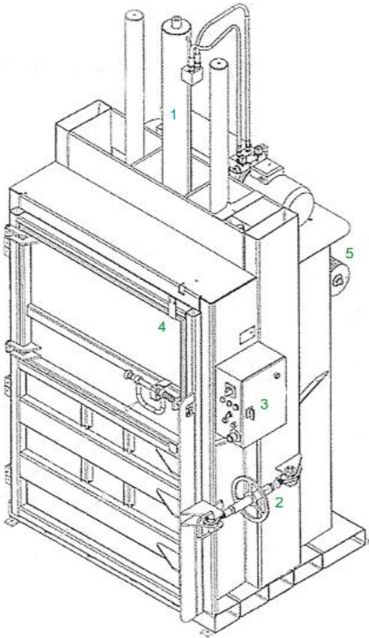
1 - Vérin double effet à tige chromée dur et 2 colonnes de guidage
